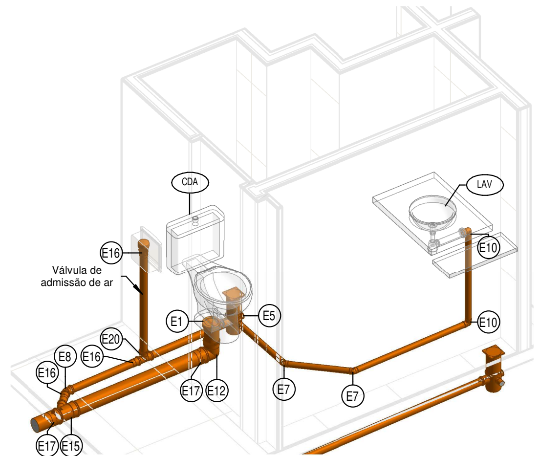
PERSPECTIVA 05 - ESGOTO
